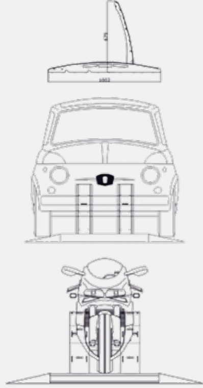
Ön-Arka Görünümü
